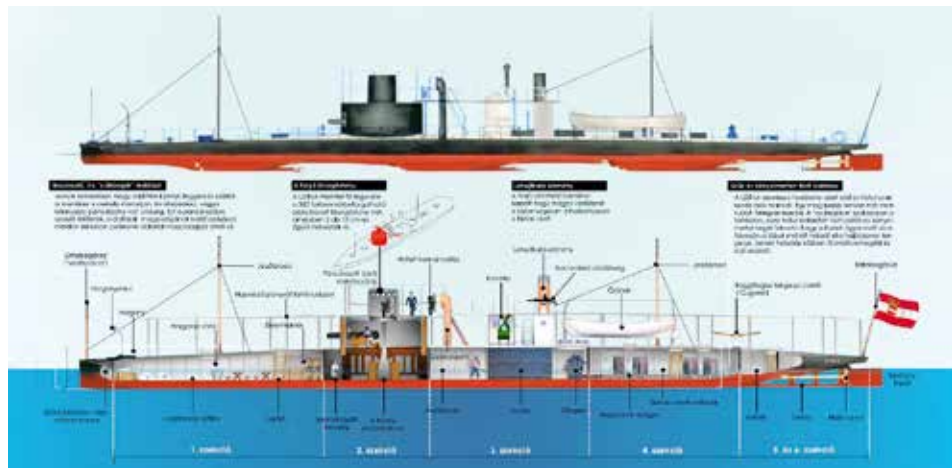
A LEITHA/LAJTA monitor hosszmetsete
