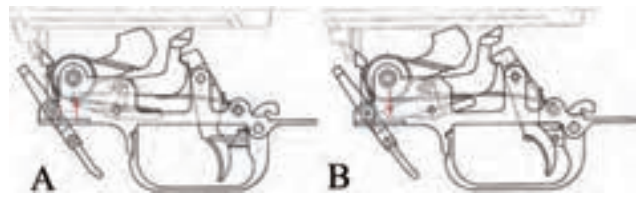
21. ábra. A tűzváltó és működési módjai
