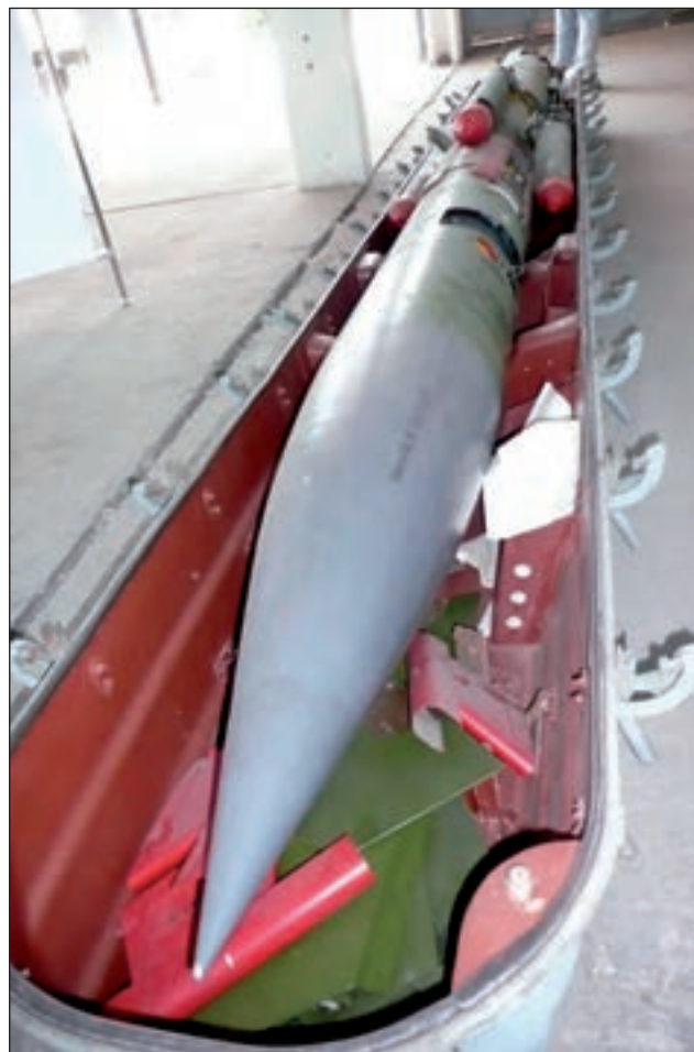
7. ábra. 3M9 típusú Kub légvédelmi rakéta a tartós tárolásra alkalmazott konténerben. A képen a rakéta tantermi változata látható, amelyen kialakított nyílásokon a belső szerkezeti elemeket is tanulmányozhatták
