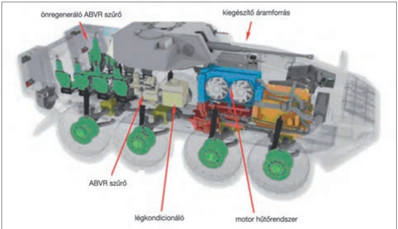
1. ábra. Kerekcs harcjármű ABVR szűrőrendszerrel
