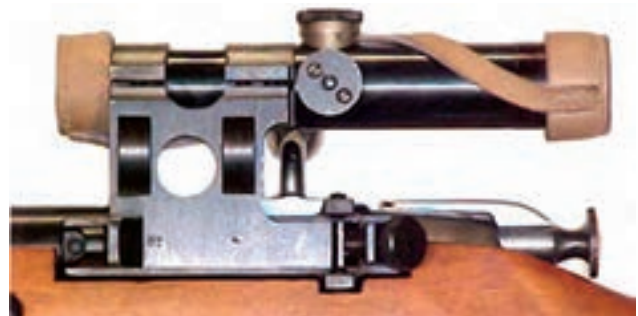
24. ábra. Az optikai irányzék
