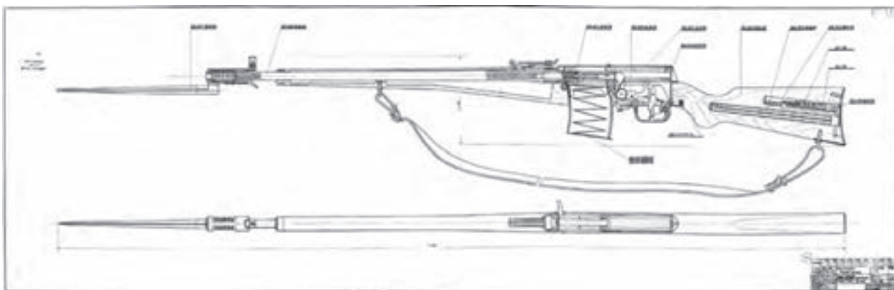
7. ábra. Kísérleti öntöltő puskára szuronyal
