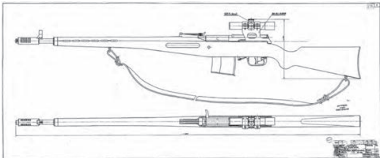
8. ábra. Kísérleti öntöltő puskára távcsővel
